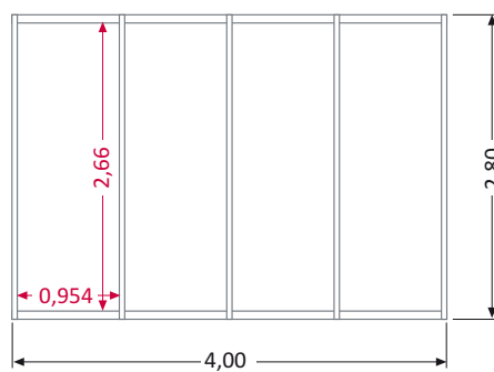
COTAS EN ROJO: MEDIDAS ÚTILES DE PANEL
