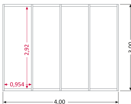
COTAS EN ROJO: MEDIDAS ÚTILES DE PANEL
