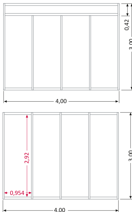
COTAS EN ROJO: MEDIDAS ÚTILES DE PANEL
